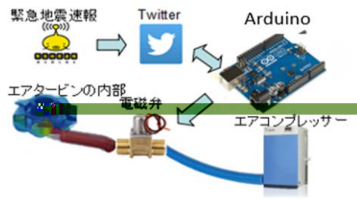
停止システムの構成
